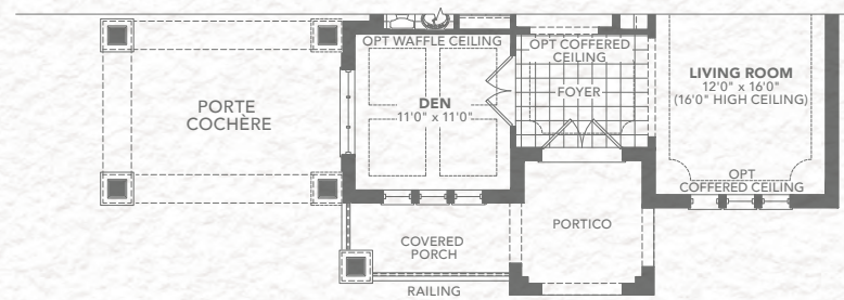
ELEVATION B
