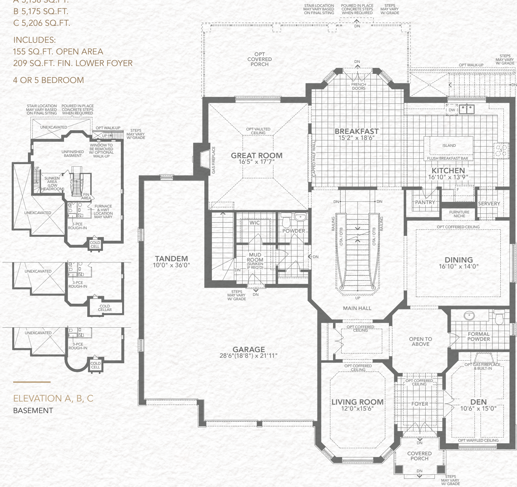
ELEVATION B
